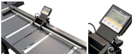
MRA - manueller Materialanslag mit digitalem Display
